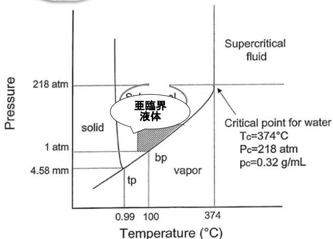
温度による水の状態の変化
