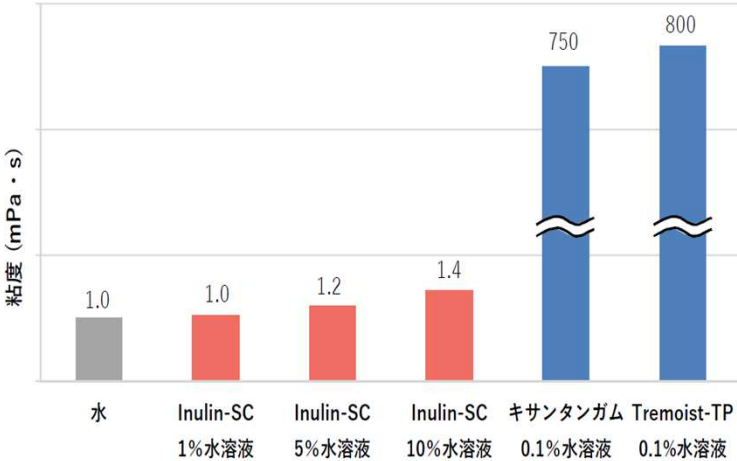
多糖類を配合した際の粘度変化 (20°C)
