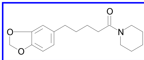
テトラヒドロピペリンの構造式
